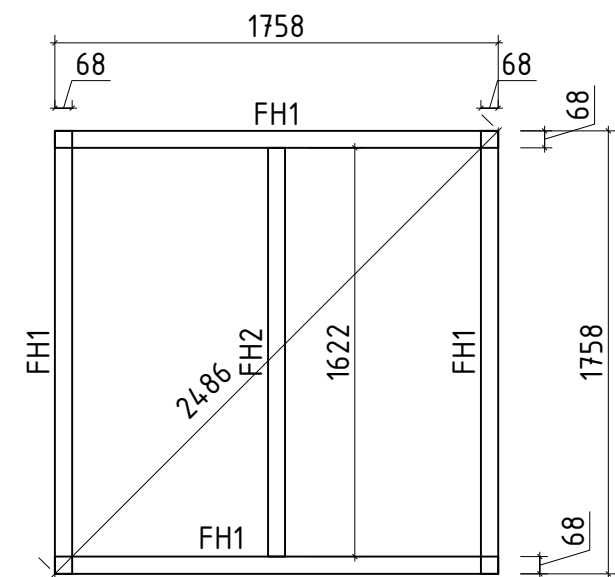
Alustalade plaan, Lagerholzplan, Foundation beams
